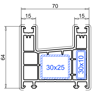
Marco deslizante 64 mm ref. 105.351 Refuerzo 113.002 (30x25) Refuerzo 113.020 (30x10)
