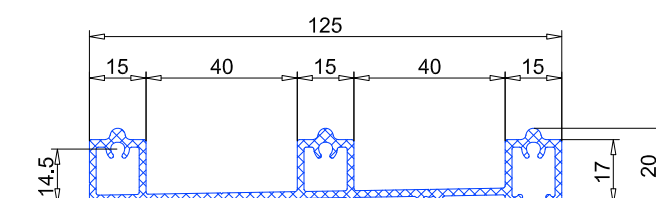
Solera de aluminio 3 carriles ref. 104.045 Cortavientos 112.230
