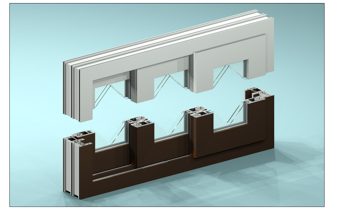
Esquema 3 carriles 3-fojas, todas deslizantes
