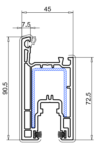
Hoja deslizante 90,5 mm ref. 105.327 Refuerzo 113.043.2 Refuerzo 113.035.2
