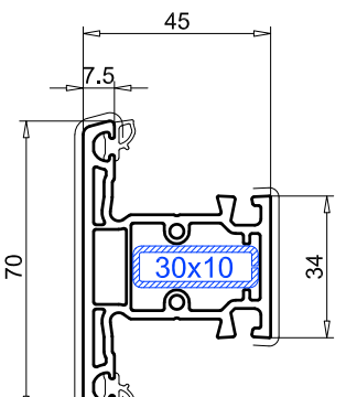
Travesaño hoja deslizante ref. 105.326 Refuerzo 113.020 Plantilla 146.016.1
