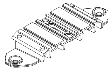
Portajuntas central ref. 109.639.2 Burlate 112.462 Color: blanco y negro
