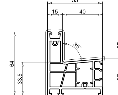
Suplemento marco tercer carril ref. 105.352
