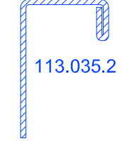
Hoja deslizante 90,5 mm ref. 105.327 Refuerzo 113.043.2 Refuerzo 113.035.2
