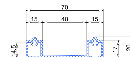
Solera de aluminio 2 carriles ref. 104.044 Cortavientos 112.230
