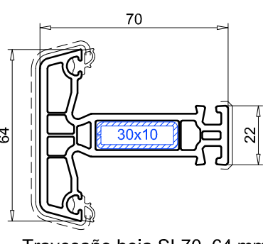
Travesaño hoja SL70, 64 mm ref. 102.237 Refuerzo 113.020 Tope metal. 106.204.1 Plantilla 146.020.0
