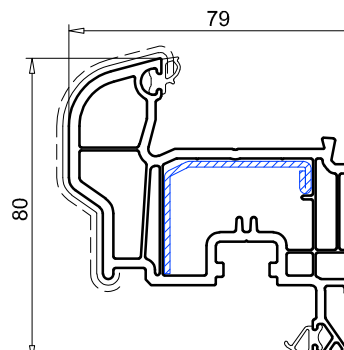
Hoja semialineada SW 80 mm ref. 103.236 Refuerzo 113.059 (sólo blanco) Refuerzo 113.294 (blanco y foliado) Refuerzo 113.295 (Paralela, plegable)
