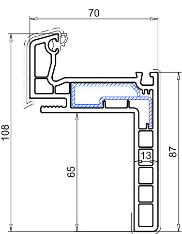
Marco renov SL70, 108 mm ref. 111.208 Refuerzo 113.312 Angulo 40/30 111.007 Angulo 80/60 111.016
