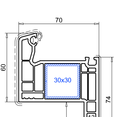
Marco con solape SL70, 67 mm ref. 101.218 Refuerzo 113.025
