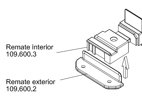
Remate interior 109.600.3 Remate exterior 109.600.2 Remate batiente 2 piezas para 102.234 ref. 109.600 Blanco, marrón y caramel
