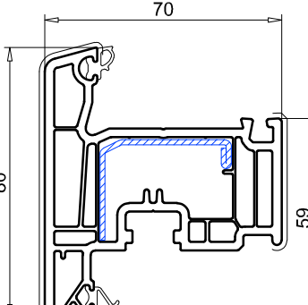
Hoja SL70 ap. exterior 80 mm ref. 103.228 Refuerzo 113.059 (sólo blanco) Refuerzo 113.294 (blanco y foliado) Refuerzo 113.295 (Plegable)
