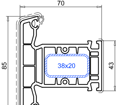
Travesaño atornillable SL70, 85 mm ref. 102.241 Refuerzo 113.272 Tope metal. 106.300.1 Zapata 106.005 Plantilla 146.020.0 (para 106.200.1) Plantilla 146.020.5 (para 106.005)
