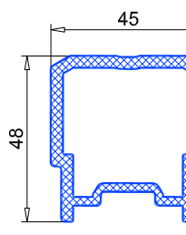
Refuerzo alu ref. 115.003 Para hojas 103.241/242/273
