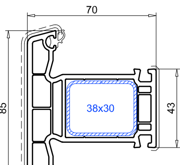
Travesaño SL70, 85 mm ref. 102.218 Refuerzo 113.271 Tope metal. 106.300.1 Pieza estanqueidad 106.086 Plantilla 146.020.0
