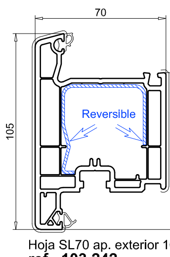
Hoja SL70 ap. exterior 105 mm ref. 103.242 Refuerzo 113.270 (sólo blanco) Refuerzo alu. 115.003 (sólo pivotante) Refuerzo 113.368.2 (blanco y foliado)
