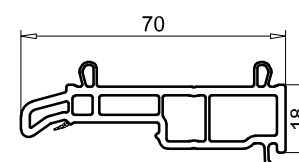
Adaptador fijos c/marco ref. 104.429 Gris/ Negro
