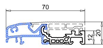
Solera PC 70 mm ref. 104.427 Alu. EV1 plata/PVC Gris Alu. EV1 plata/PVC Negro
