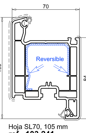
Hoja SL70, 105 mm ref. 103.241 Refuerzo 113.270 (sólo blanco) Refuerzo alu. 115.003 (sólo pivotante) Refuerzo 113.368.2 (blanco y foliado)
