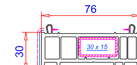
Ensanche 30 mm Ref. 114.053 Refuerzos: 113.055
