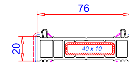
Unión de marcos 26 mm Ref. 116.230 Refuerzos: 113.028
