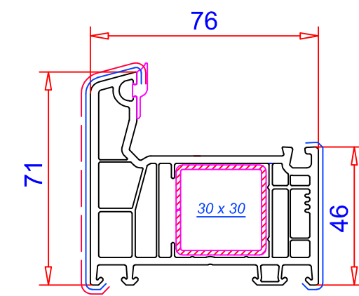
Marco DJ 71mm / Ref. 101.353 Refuerzos: 113.025 / 113.025.2 / 113.025.3
