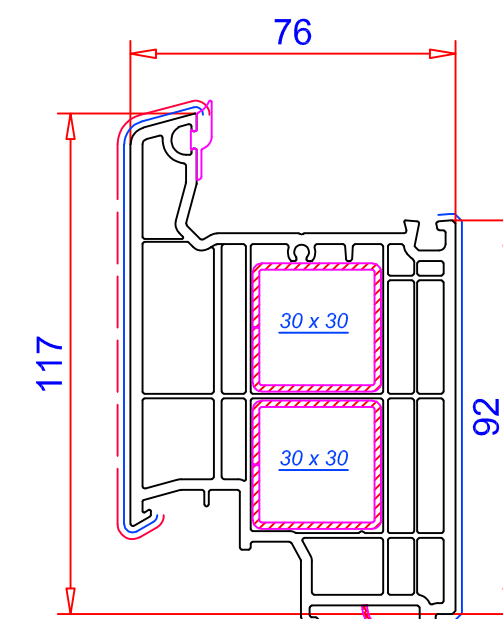
Zócalo 117 mm / Ref. 105.402 Refuerzos: 113.025 / 113.025.2 / 113.025.3
