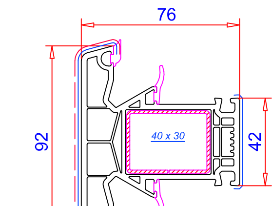
Travesaño JC 92mm / Ref. 102.350 Refuerzos: 113.001 / 113.001.3 Refuerzo / puerta: 113.367 Pieza de estanqueidad: 106.430 Tapones JC: 106.373 Pieza unión: 106.420.1 Plantilla: 146.032.1
