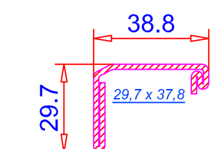
Refuerzo 29,7 x 38,8 mm Ref. 113.294.2 para 103.381
