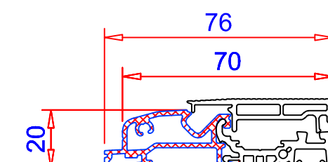
Solera SL76 Ref. 104.530 Aluminio anodizado plateado / PVC gris claro Aluminio anodizado plateado / PVC negro
