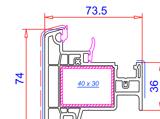
Batiente 74mm / Ref.: 102.356 Refuerzos: 113.001 / 113.001.3
