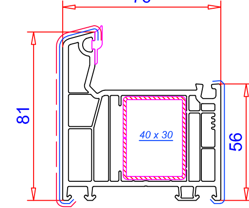
Marco DJ 81mm / Ref. 101.354 Refuerzos: 113.001 / 113.001.3 113.367 / puerta
