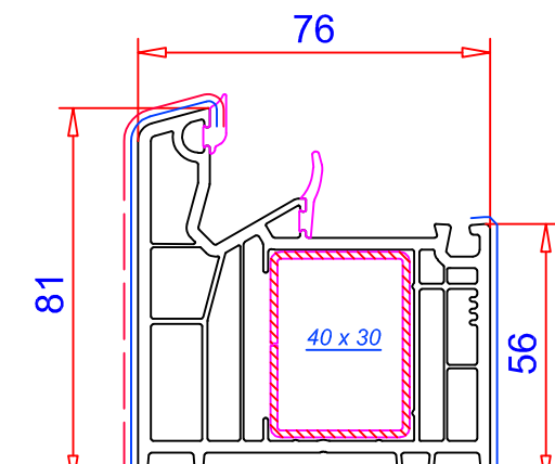
Marco JC 81mm / Ref. 101.351 Refuerzos: 113.001 / 113.001.3 113.367 / puerta
