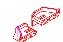
Tapones JC Ref. 106.373 para 102.350 / 102.351 Material: TPE SD 333 50 A Color: gris plateado / negro
