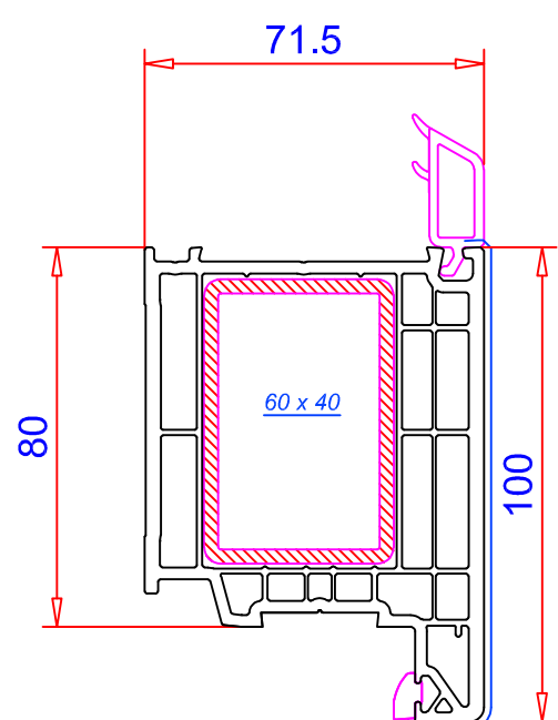
Hoja panel 125 mm / Ref. 105.403 Refuerzo: 113.011.3 Refuerzo esp: 113.011.5 Topes soldables: 141.530 Atornillador para 141.530: 141.528
