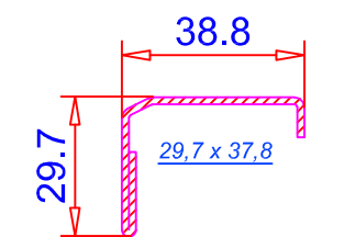
Refuerzo 29,7 x 38,8 mm Ref. 113.292 para 103.381
