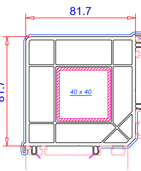
Esquinero 90° de 82 mm Ref. 107.264 Refuerzo: 113.281.2
