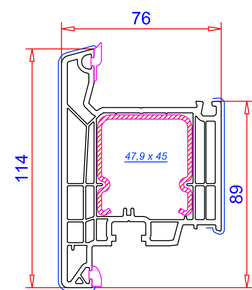
Hoja 114 mm / Ref. 103.385 Refuerzo: 113.368.2 Topes soldables: 141.531 Atornillador para 114.531: 141.528 Refuerzo: 113.270 Refuerzo alu.: 115.003
