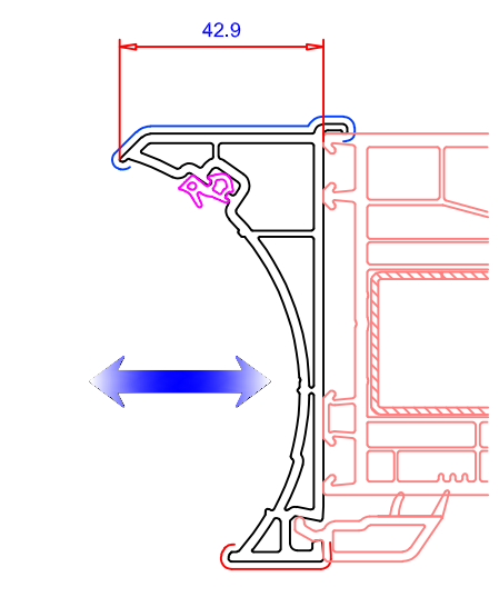
Acoplamiento esquinero reg. Ref. 116.215.2 Junquillo 107.261 Junta 112.253
