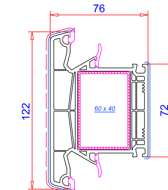
Travesaño JC 122mm / Ref. 102.351 Refuerzos: 113.011 / 113.011.2 / 113.011.3 Pieza estanqueidad: 106.431 Tapones JC: 106.373 Pieza unión: 106.422.1 Plantilla: 146.032.1
