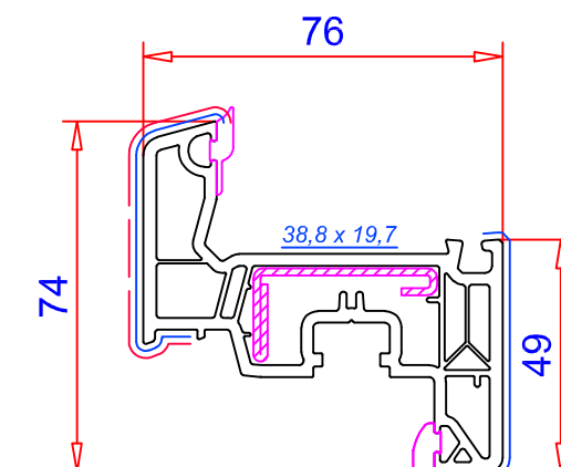
Hoja 74 mm / Ref. 103.380 Refuerzo: 113.363
